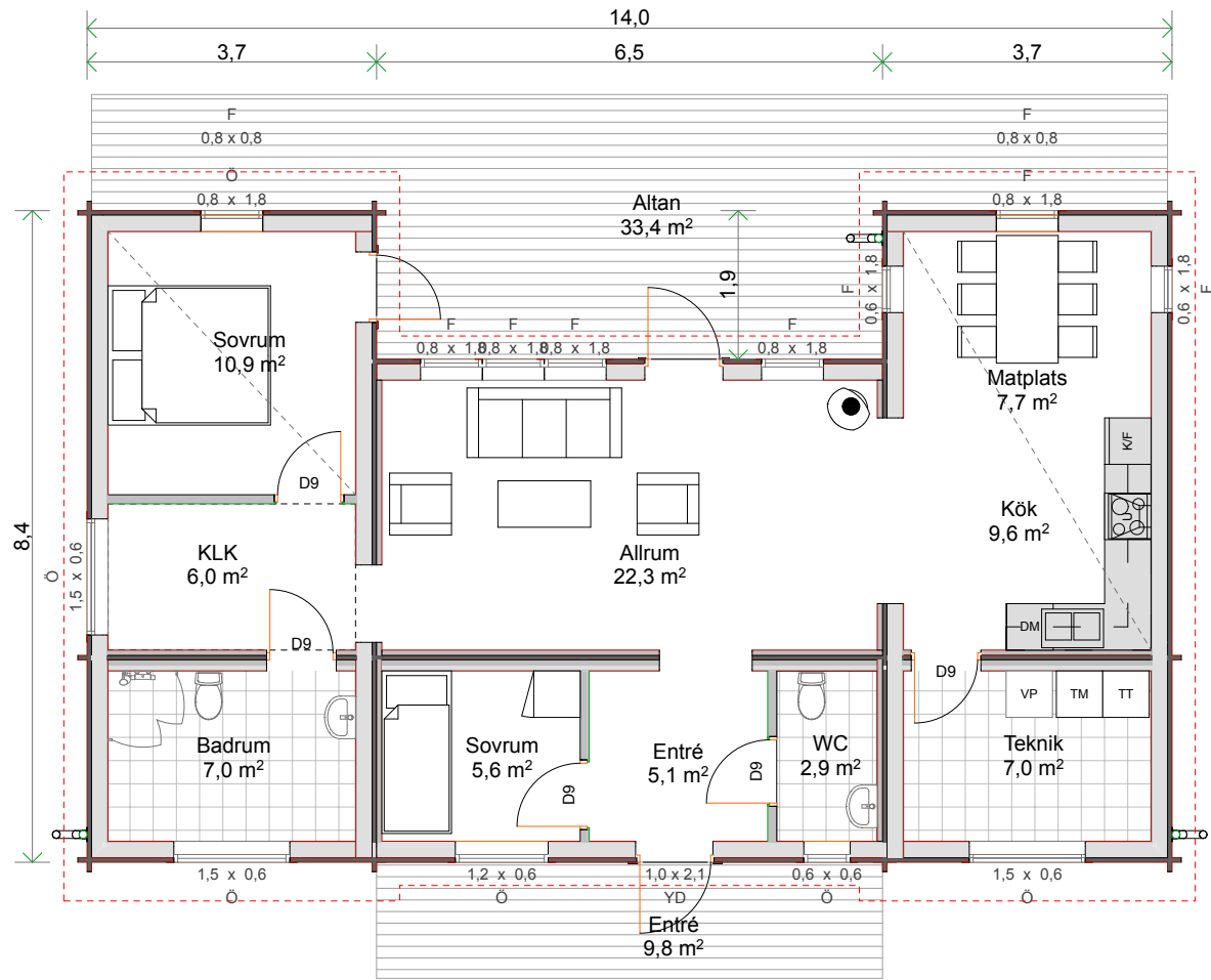
Plan 1 BYA 105,6 m 2 BOA 92,6 m 2
