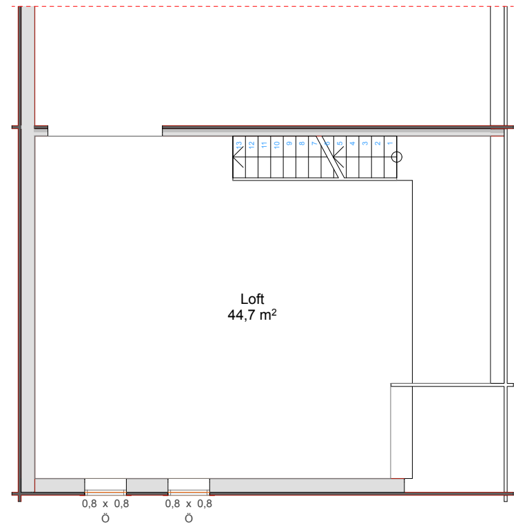
Plan 2 1:100
