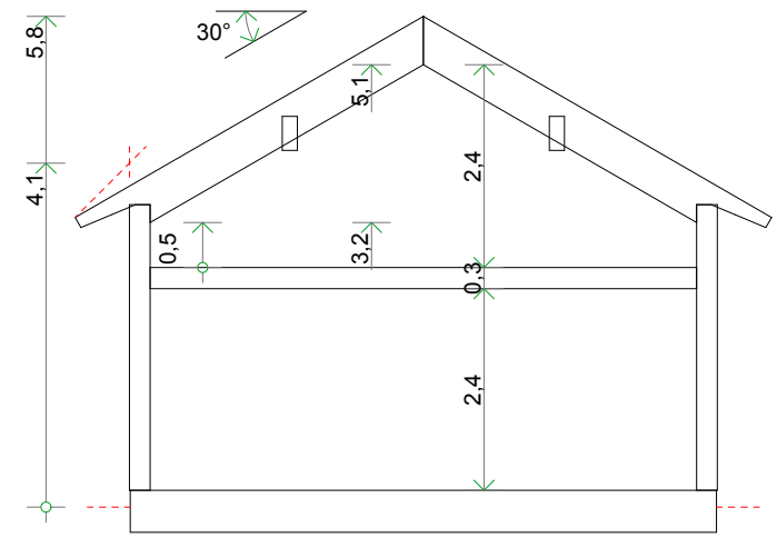
2D Sektion 1 1:100
