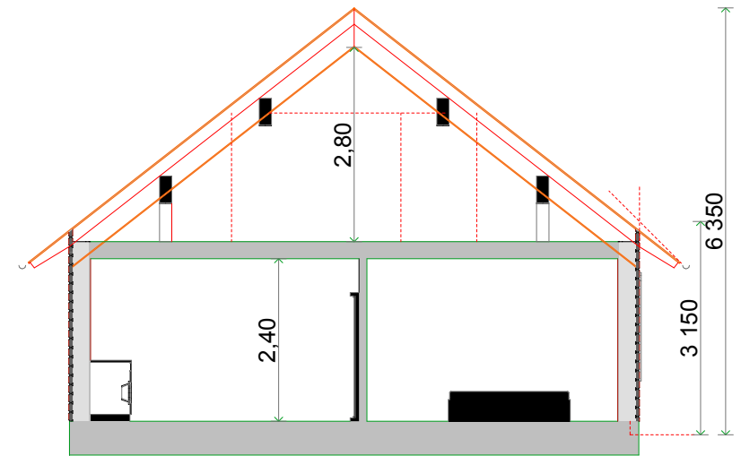
Sektion A-A 1:100
