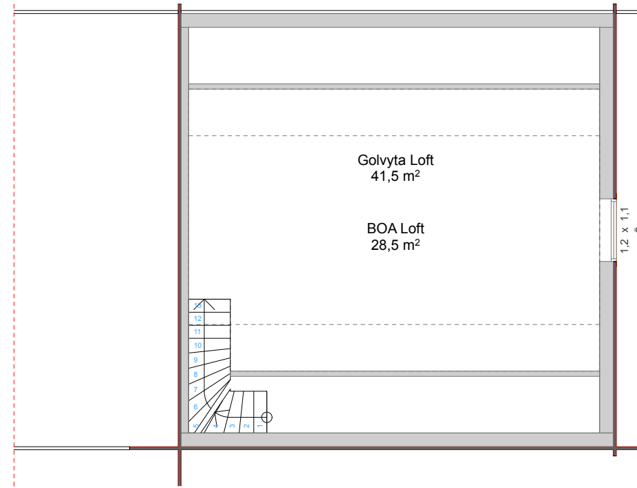
Plan 2 1:100
