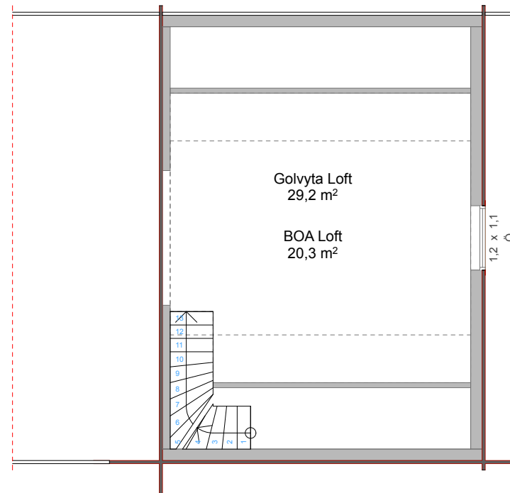
Plan 2 1:100
