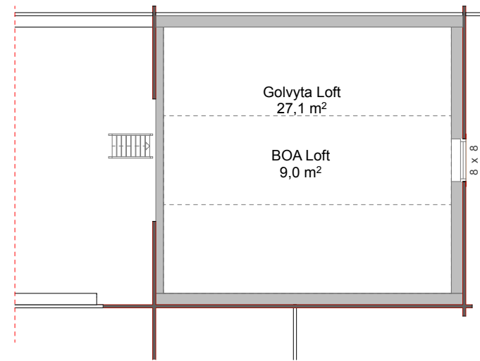
Plan 2 1:100
