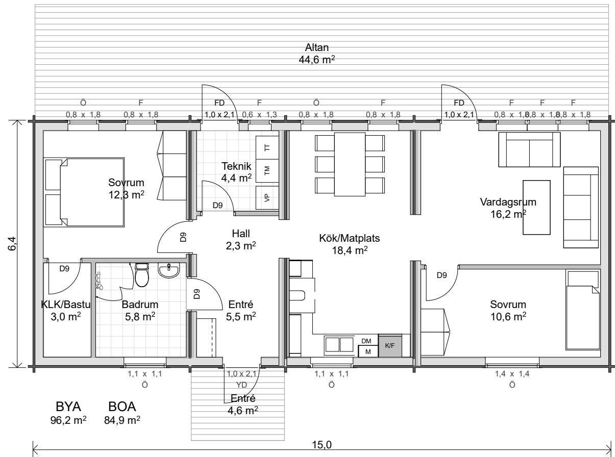
Plan 1 1:100
