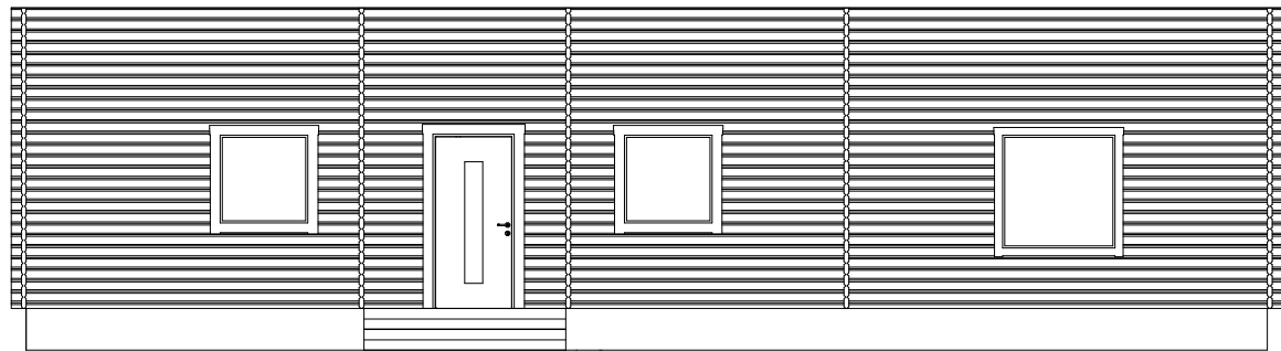
Fasad A1 1:100
