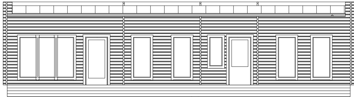
Fasad A3 1:100
