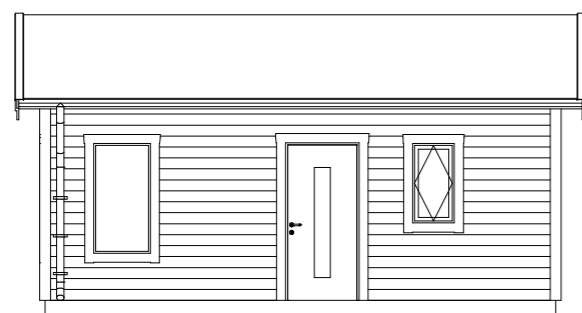
Fasad A1 1:100
