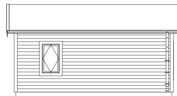
Fasad A3 1:100
