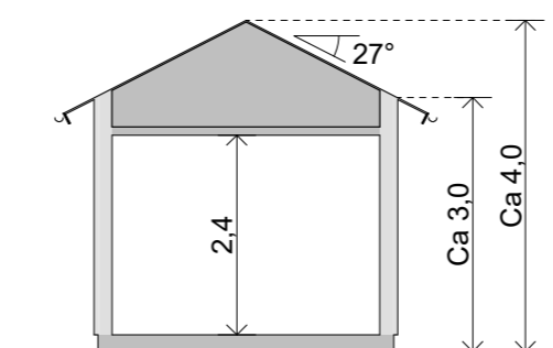
Sektion A 1:100
