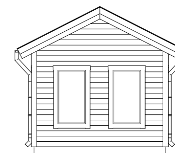
Fasad A4 1:100
