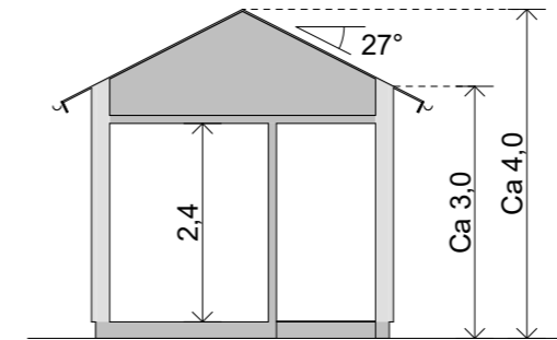
Sektion A 1:100
