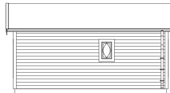
Fasad A3 1:100
