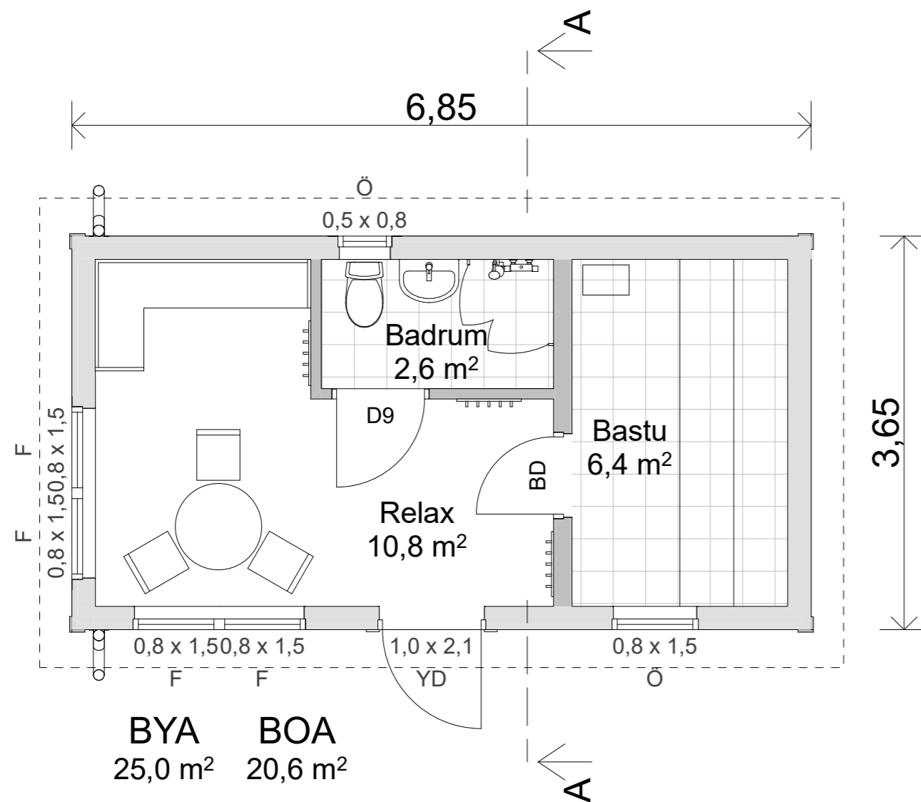
Plan 1 1:50
