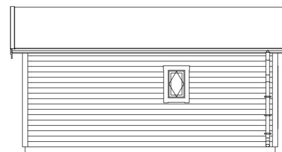
Fasad A3 1:100
