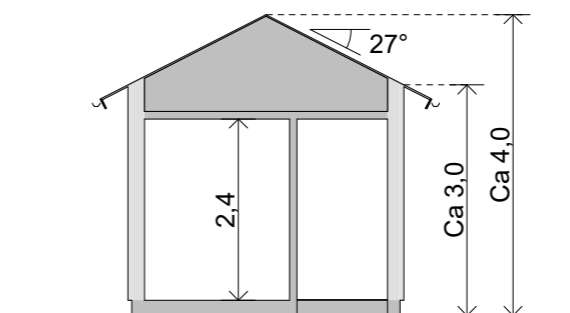
Sektion A 1:100
