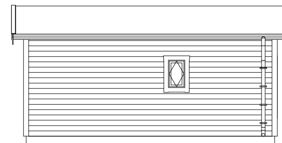
Fasad A3 1:100
