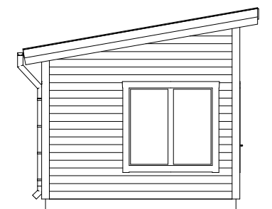
Fasad A4 1:100
