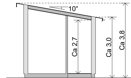
Sektion A 1:100
