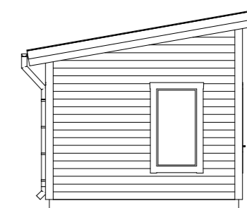
Fasad A4 1:100
