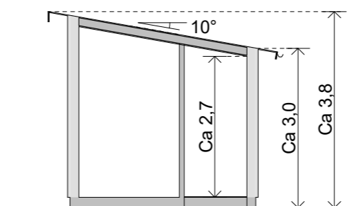
Sektion A 1:100
