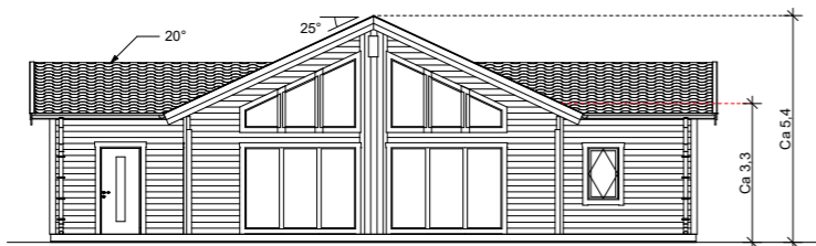
Fasad A1 1:200
