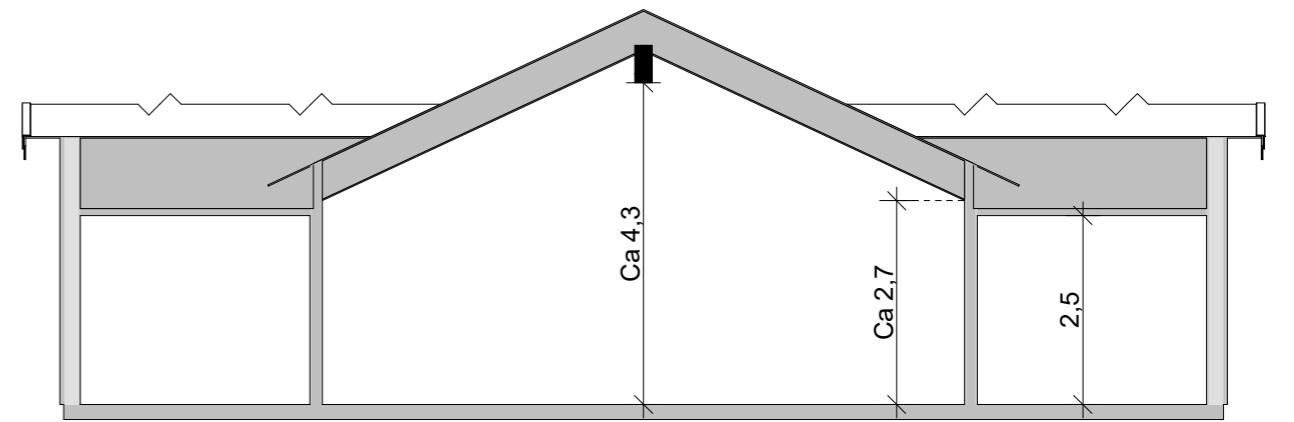
Sektion A 1:100
