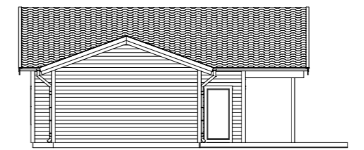
Fasad A4 1:200
