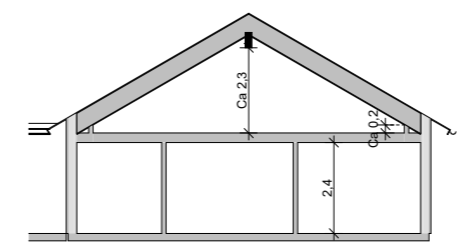
Sektion B 1:200
