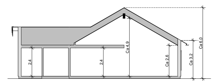
Sektion A 1:200
