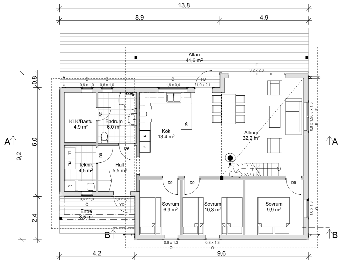
BYA 128,7 m 2 BOA 98,3 m 2 Plan 1 1:100
