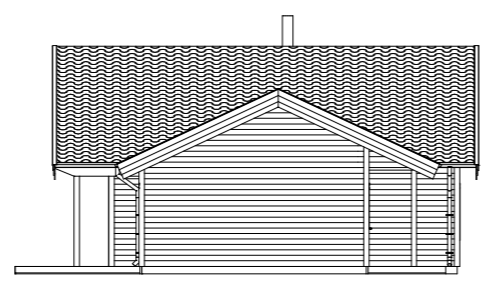
Fasad A4 1:200
