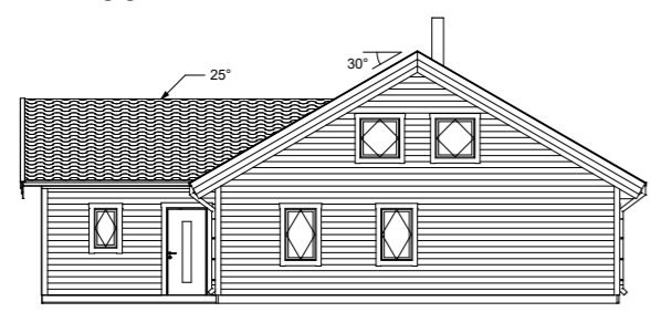
Fasad A1 1:200
