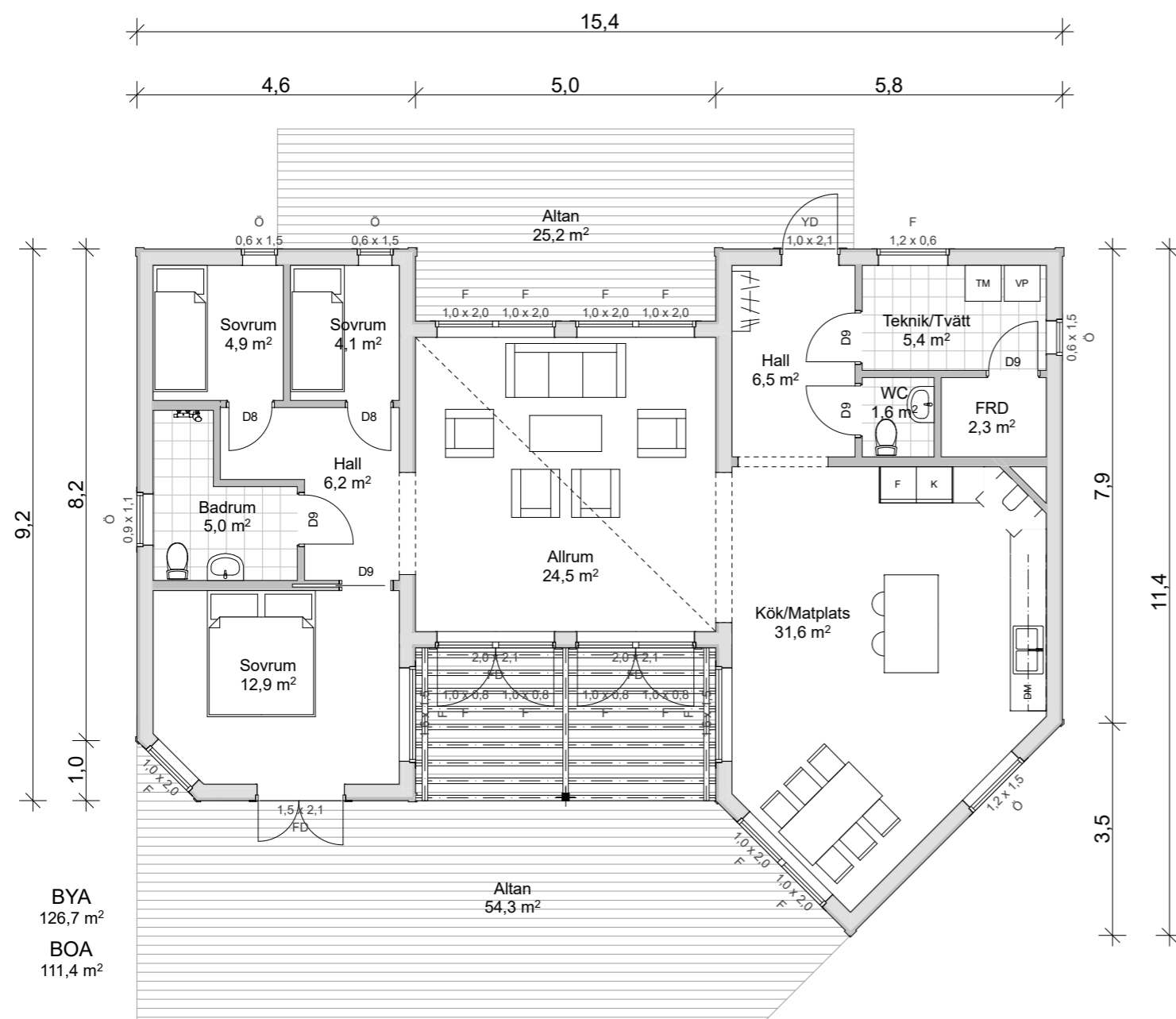
Plan 1 1:100
