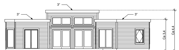
Fasad A1 1:200
