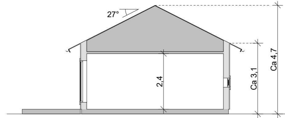
Sektion A 1:100
