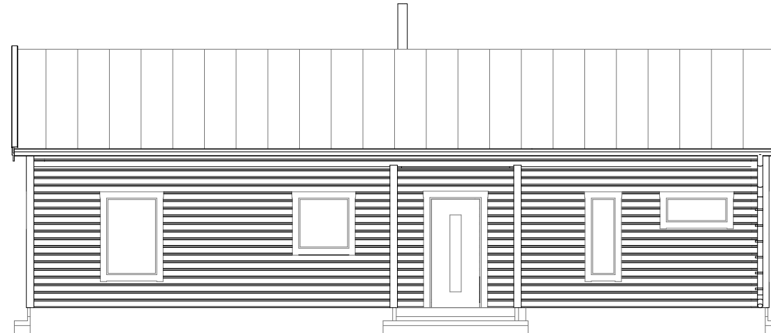
Fasad A1 1:100
