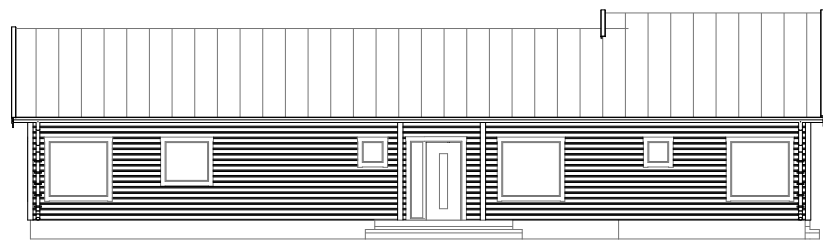
Fasad A1 1:200
