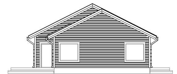
Fasad A4 1:200
