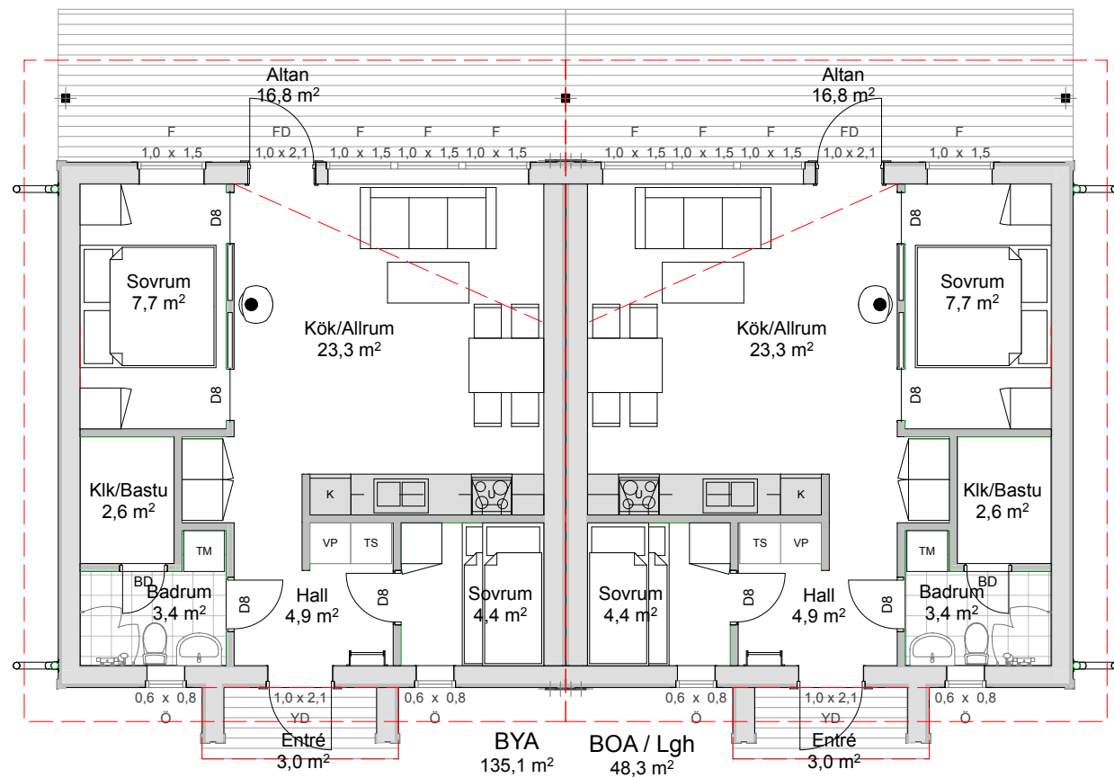
Plan 1 1:100
