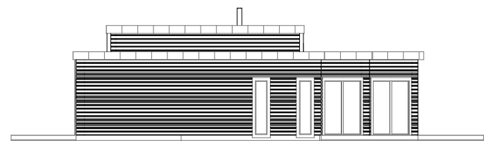
Fasad A4 1:200
