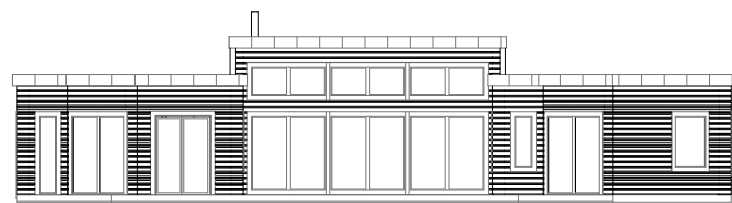
Fasad A1 1:200
