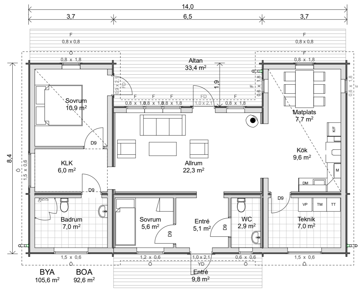
Plan 1 1:100
