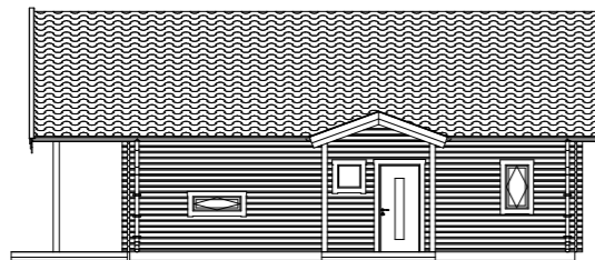
Fasad A1 1:200
