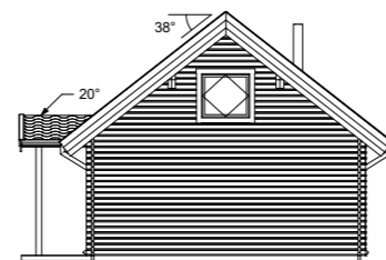
Fasad A2 1:200
