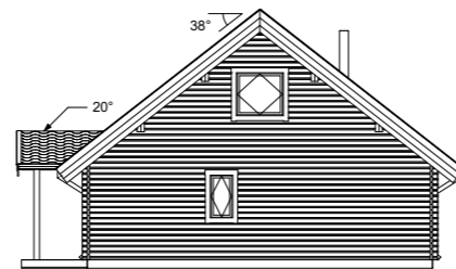
Fasad A2 1:200
