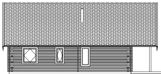
Fasad A3 1:200
