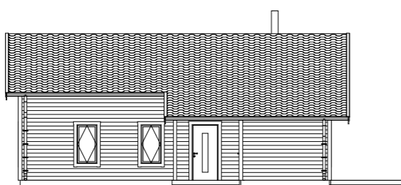
Fasad A1 1:200
