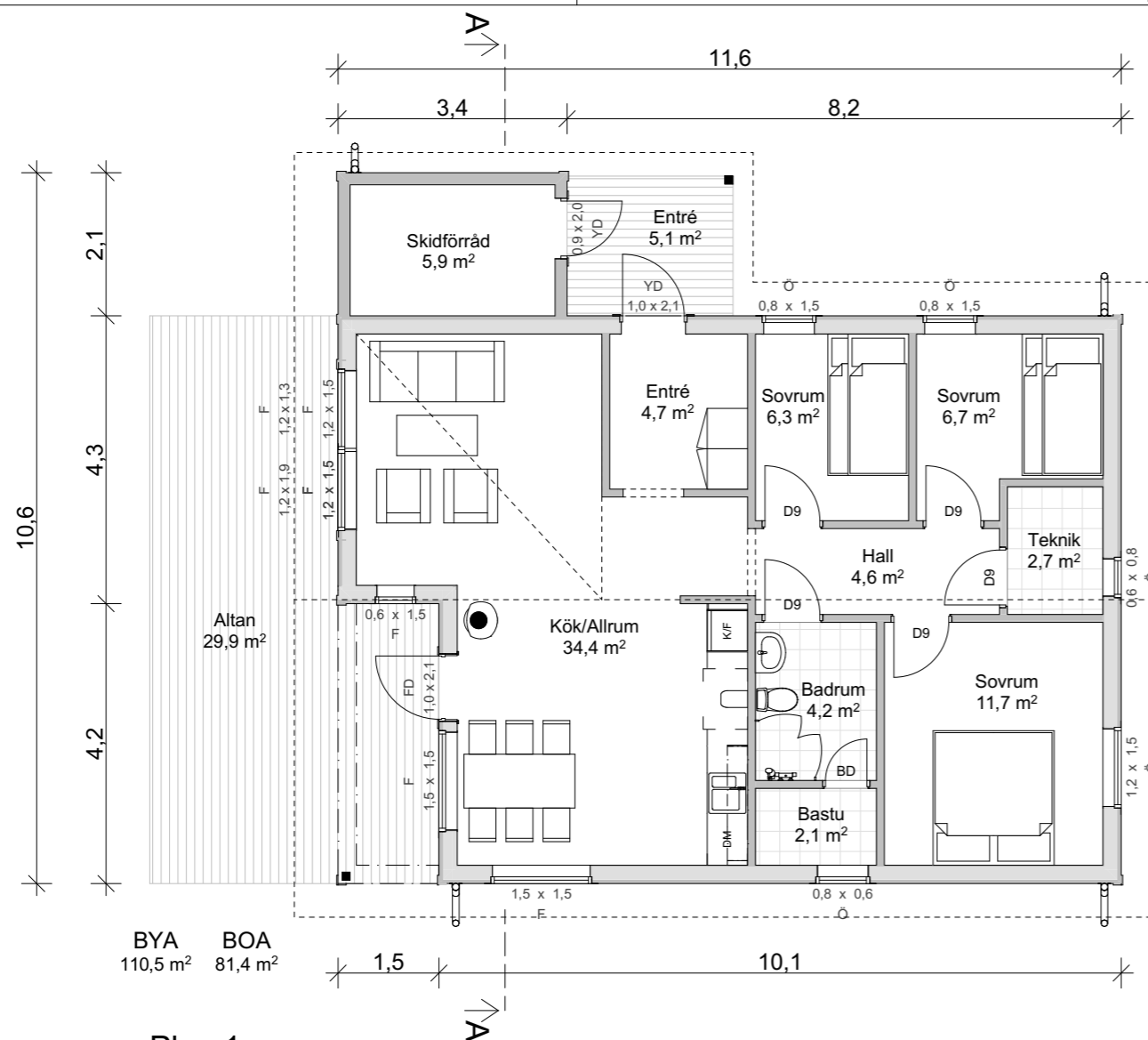
Plan 1 1:100
