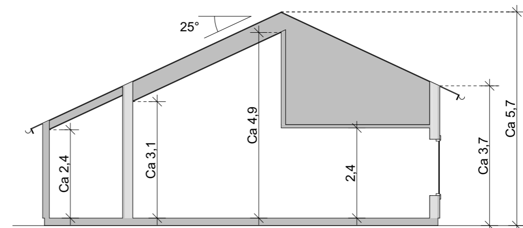
Sektion A 1:100
