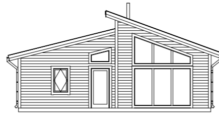
Fasad A2 1:200
