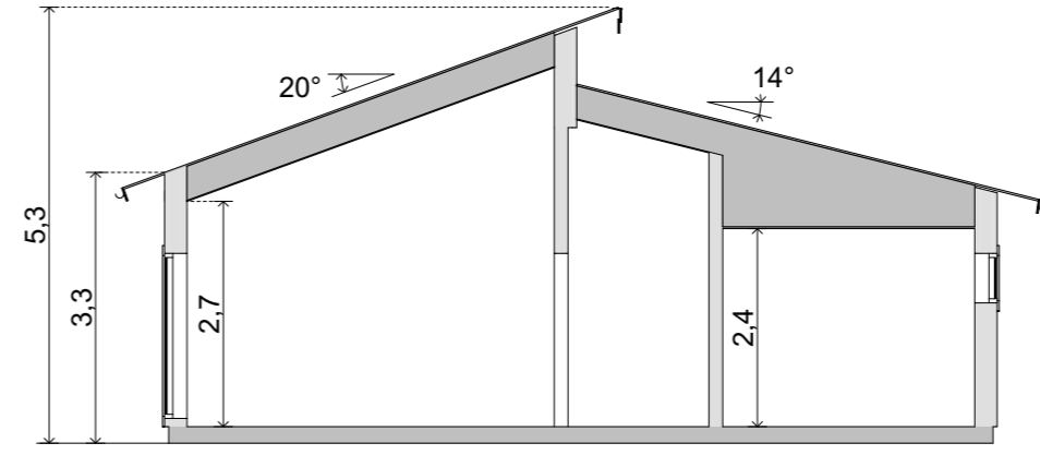
Sektion A 1:100
