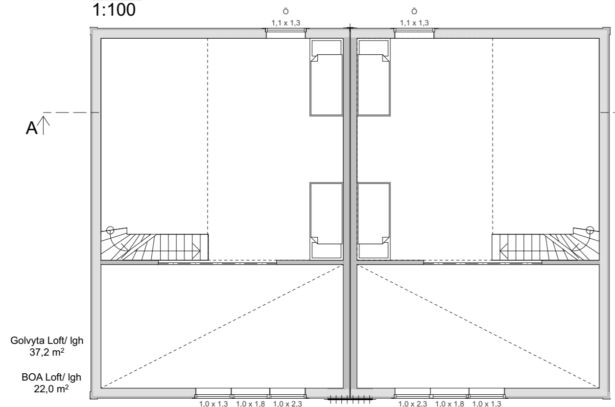
Plan Loft 1:100
