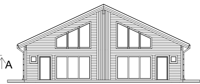
Fasad A1 1:200
