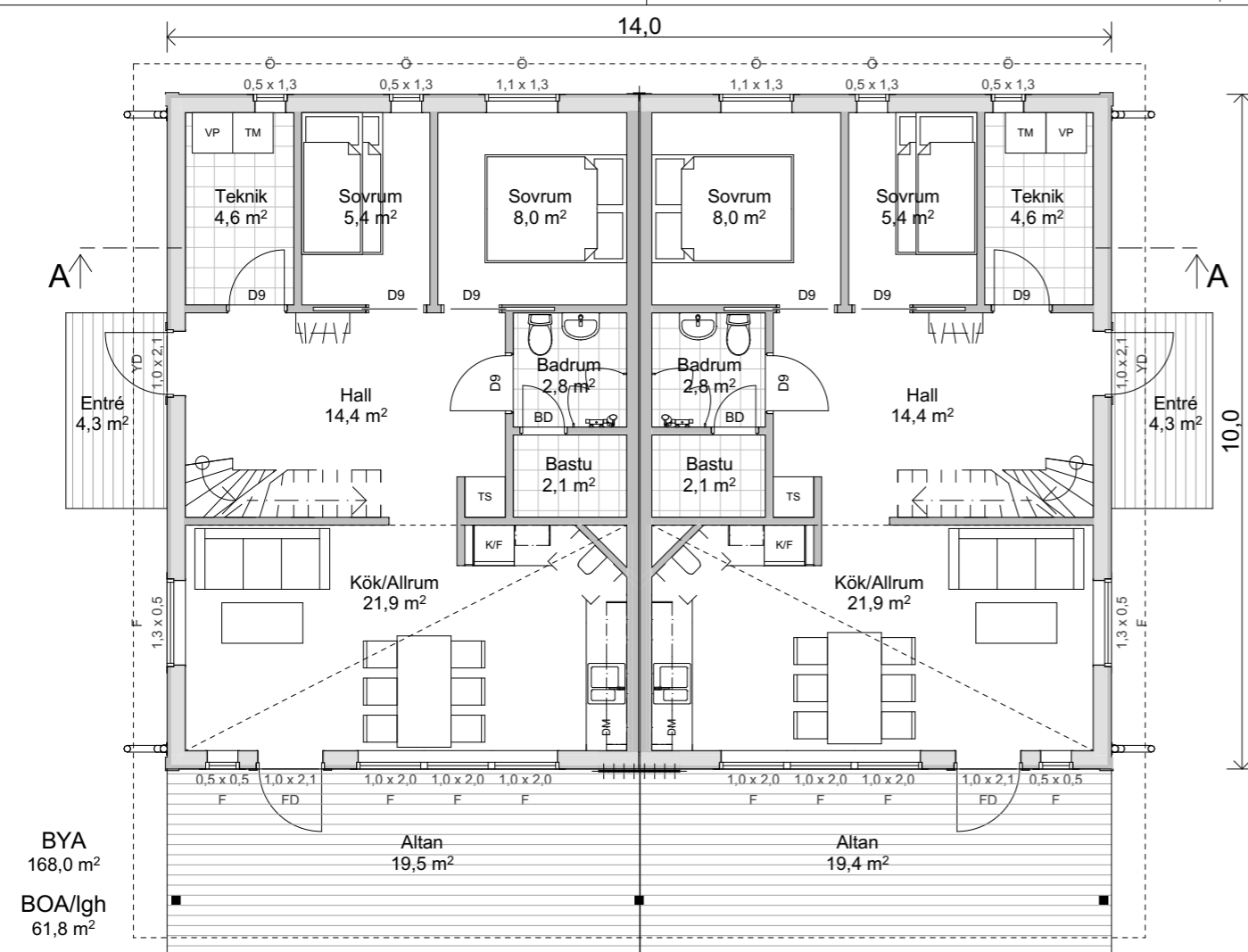
Plan 1 1:100
