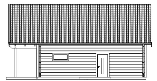
Fasad A2 1:200
