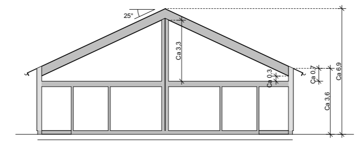
Sektion A 1:200
