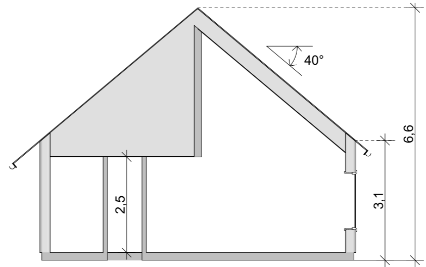
Sektion A 1:100
