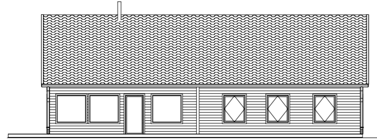
Fasad A1 1:200
