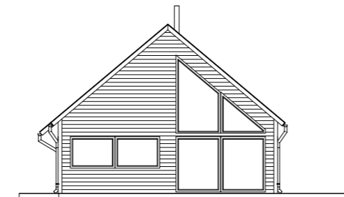
Fasad A4 1:200
