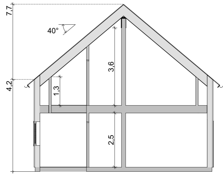
Sektion A 1:100
