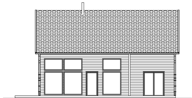
Fasad A1 1:200
