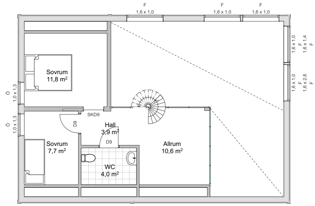
Golvyta Loft 40,3 m 2 BOA Loft 39,2 m 2 Plan 2 1:100
