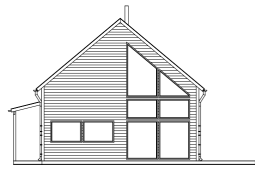
Fasad A4 1:200
