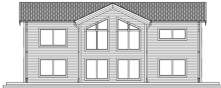
Fasad A1 1:200
