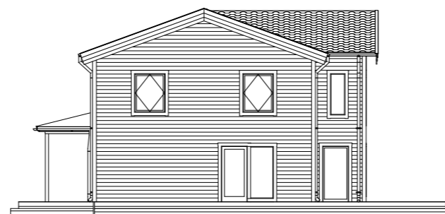
Fasad A4 1:200
