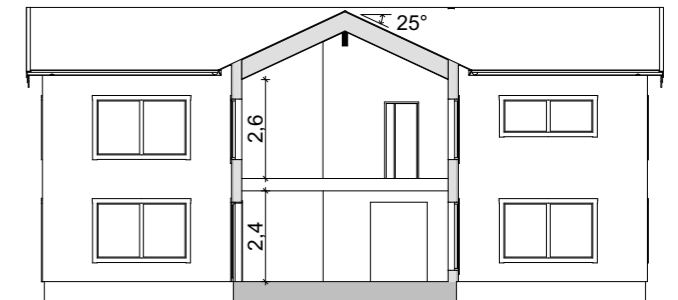
Sektion A 1:200
