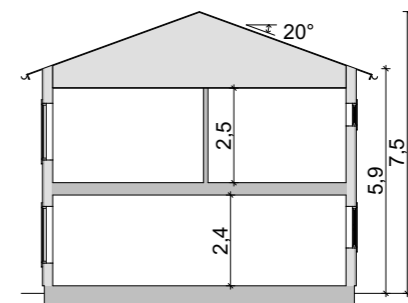
Sektion B 1:200
