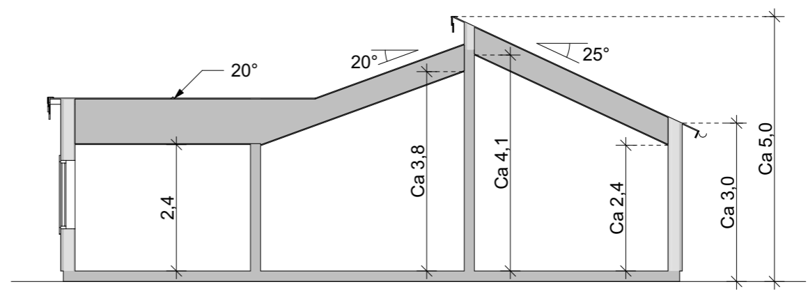
Sektion A 1:100
