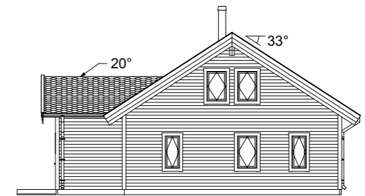
Fasad A2 1:200
