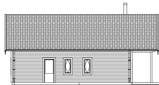
Fasad A3 1:200
