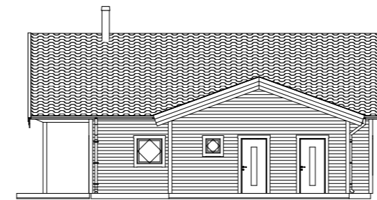
Fasad A1 1:200
