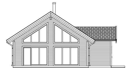
Fasad A4 1:200
