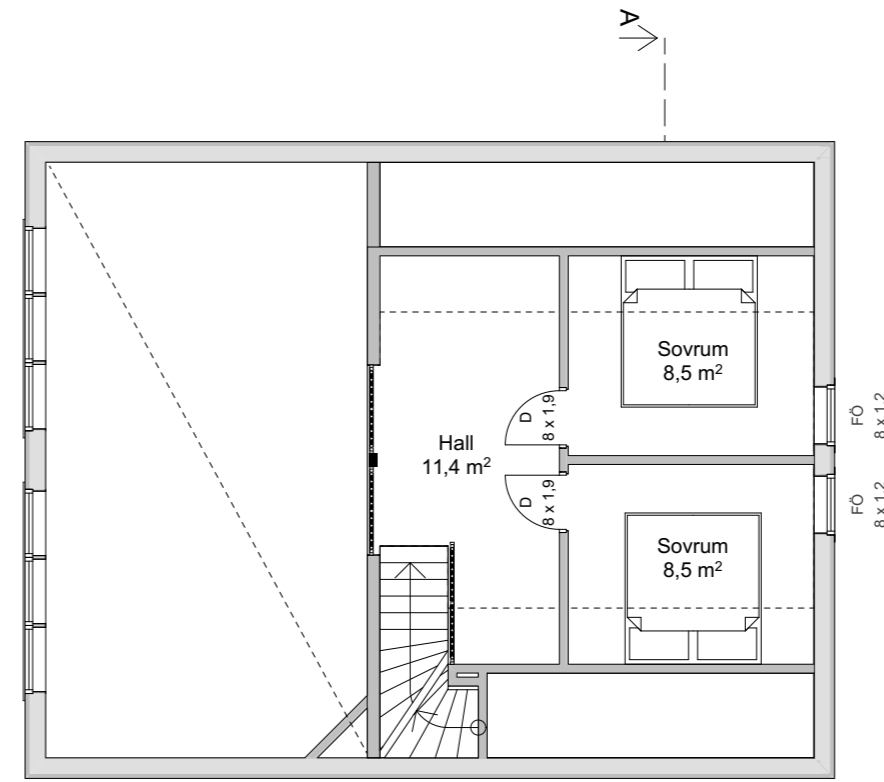
Plan Loft 1:100
