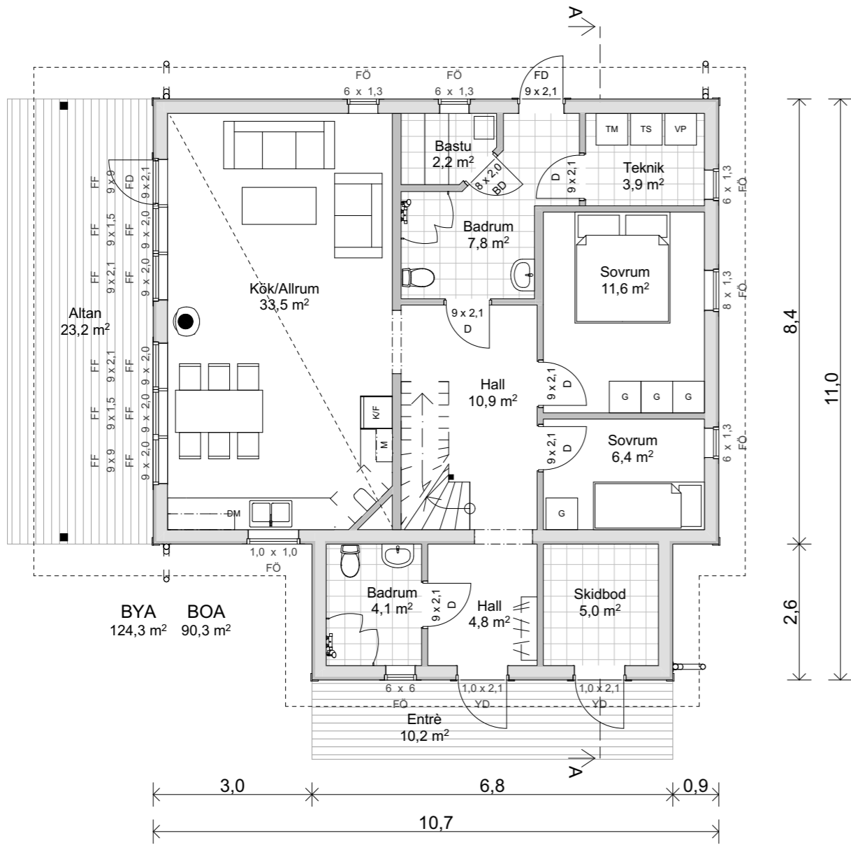
Plan 1 1:100
