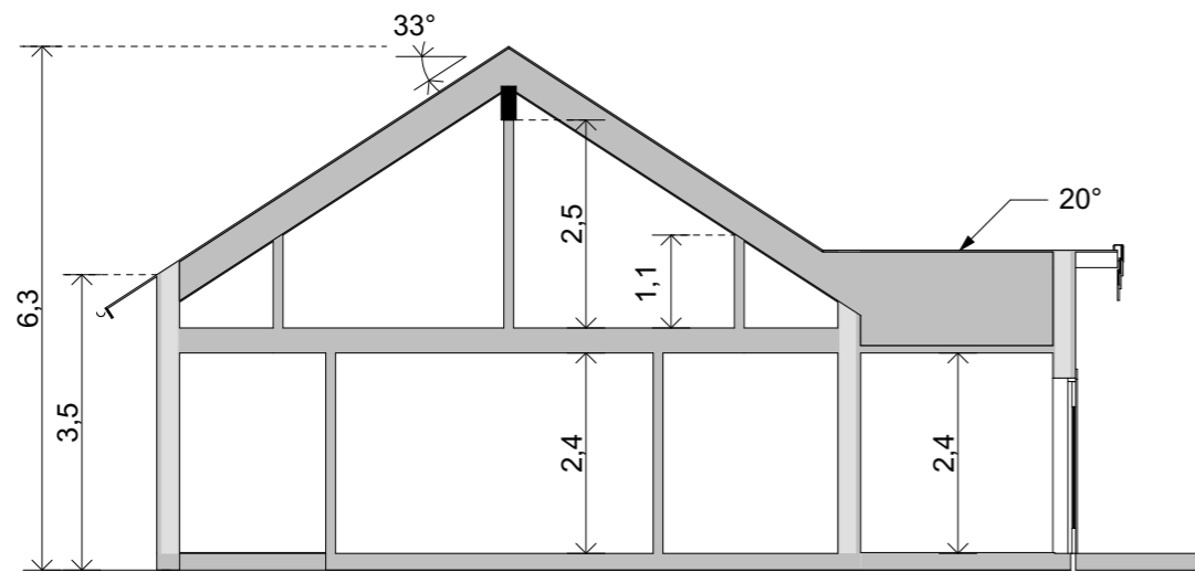
Sektion A 1:100
