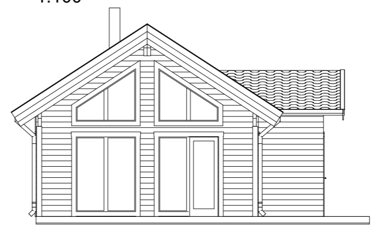
Fasad A4 1:100
