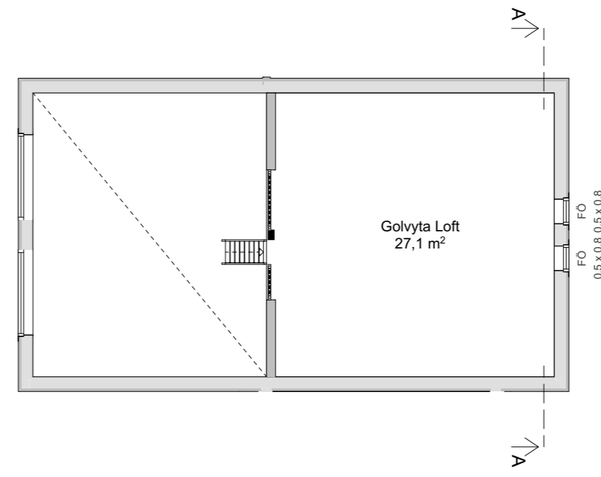
Plan Loft 1:100
