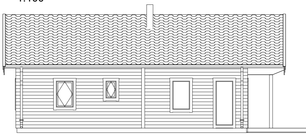
Fasad A3 1:100
