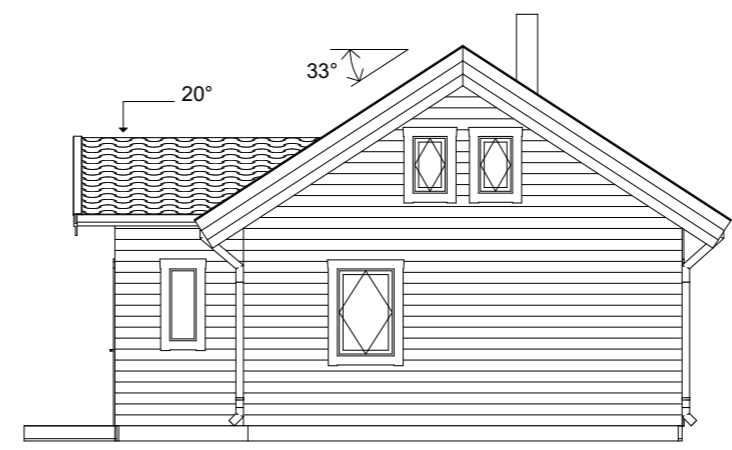
Fasad A2 1:100
