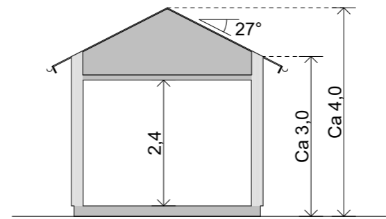
Sektion A 1:100
