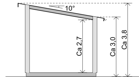
Sektion A 1:100
