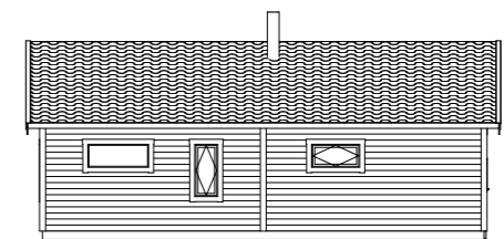
Fasad A4 1:200
