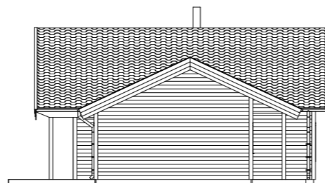
Fasad A4 1:200
