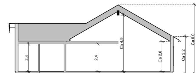
Sektion A 1:200
