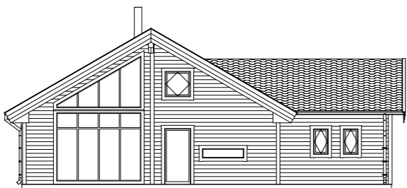
Fasad A3 1:200
