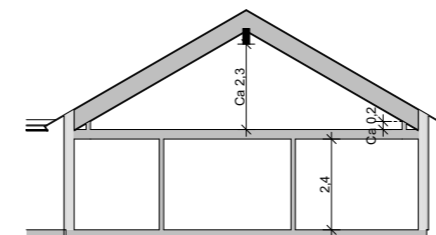
Sektion B 1:200
