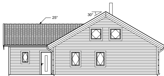
Fasad A1 1:200
