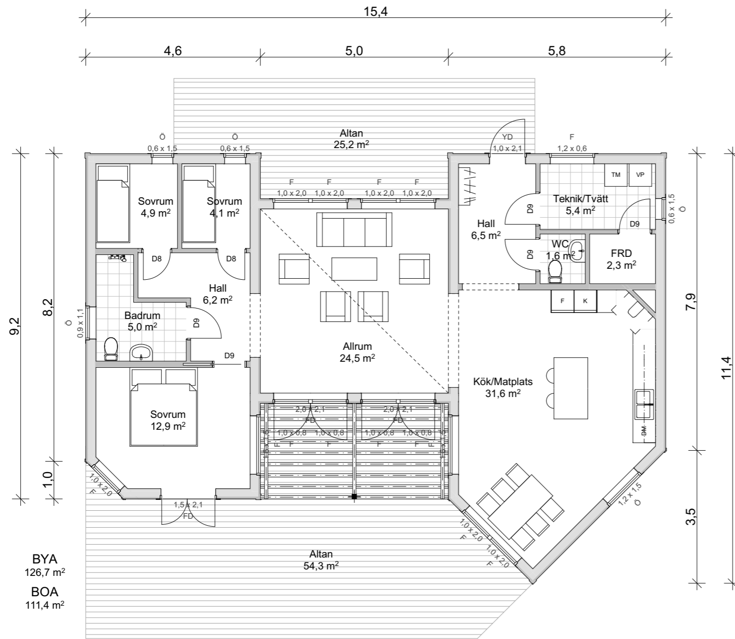
Plan 1 1:100
