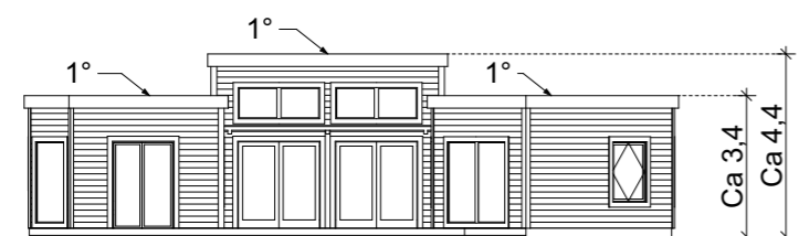
Fasad A1 1:200
