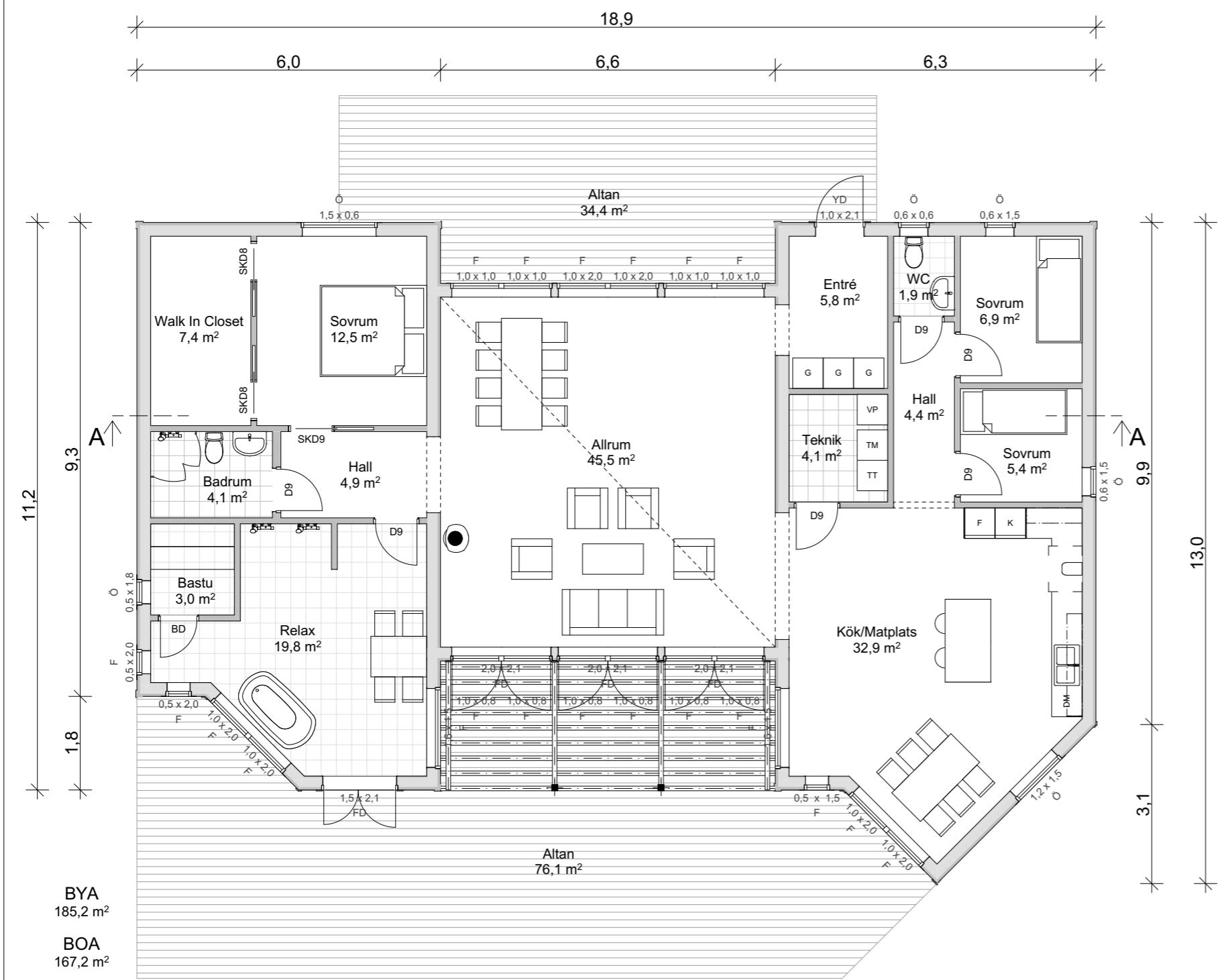
Plan 1 1:100
