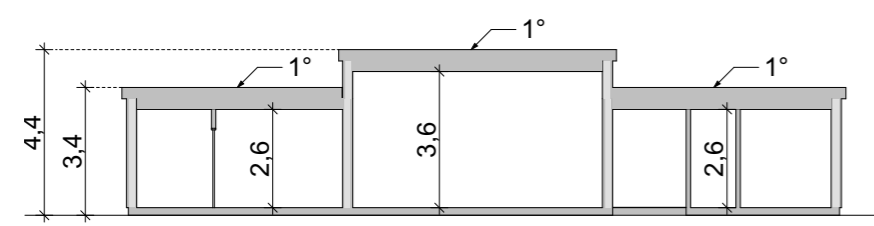
Sektion A 1:200
