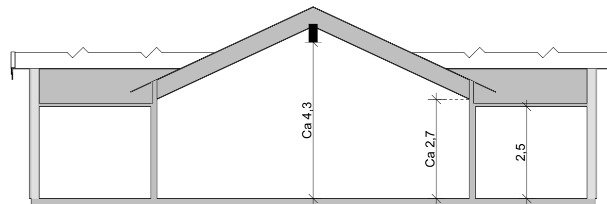
Sektion A 1:100
