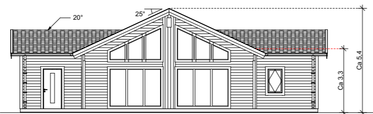
Fasad A1 1:200
