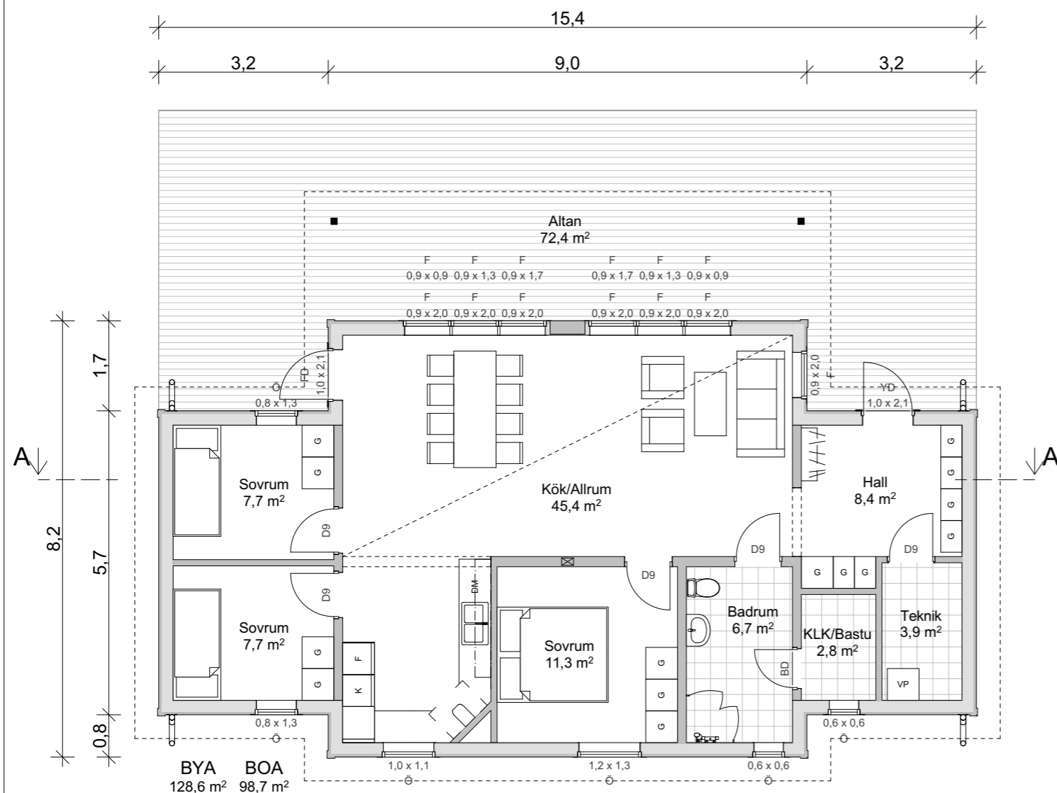
Plan 1 1:100
