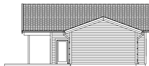
Fasad A2 1:200
