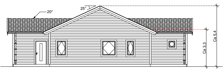
Fasad A1 1:200
