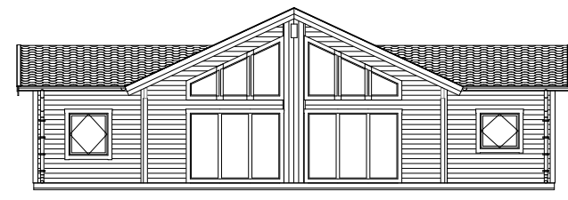
Fasad A3 1:200
