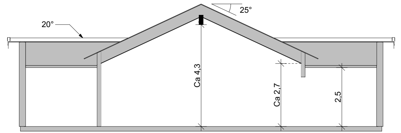
Sektion A 1:100
