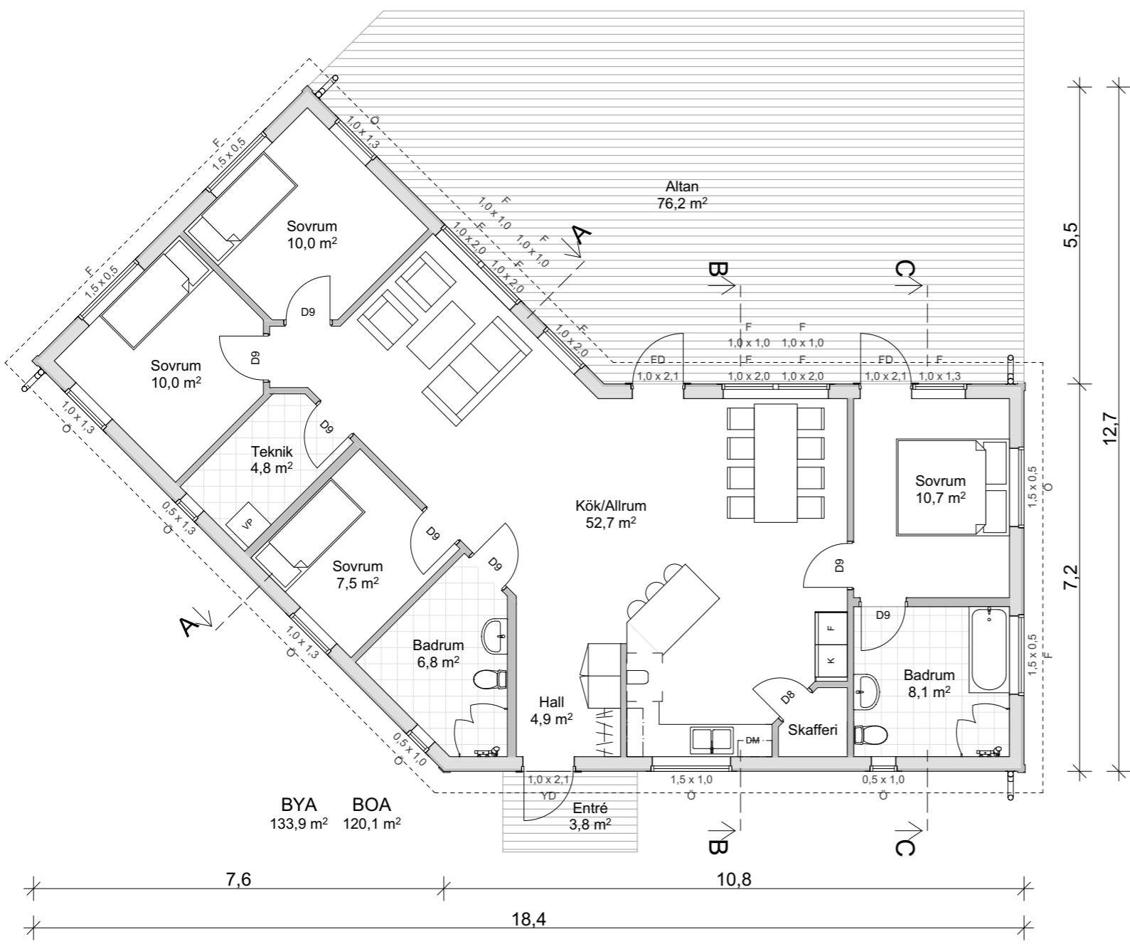
Plan 1 1:100
