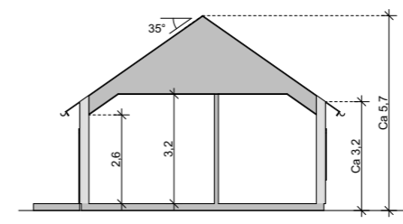
Sektion A 1:200
