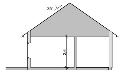
Sektion C 1:200
