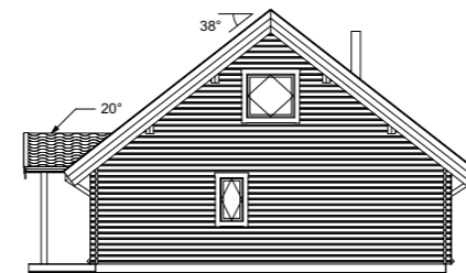
Fasad A2 1:200
