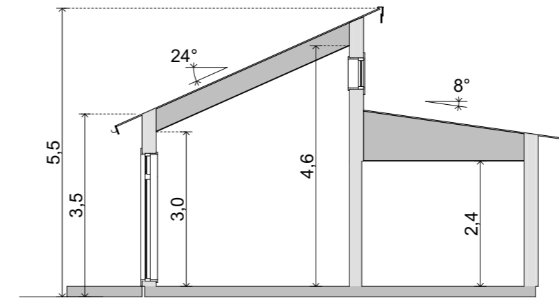
Sektion A
