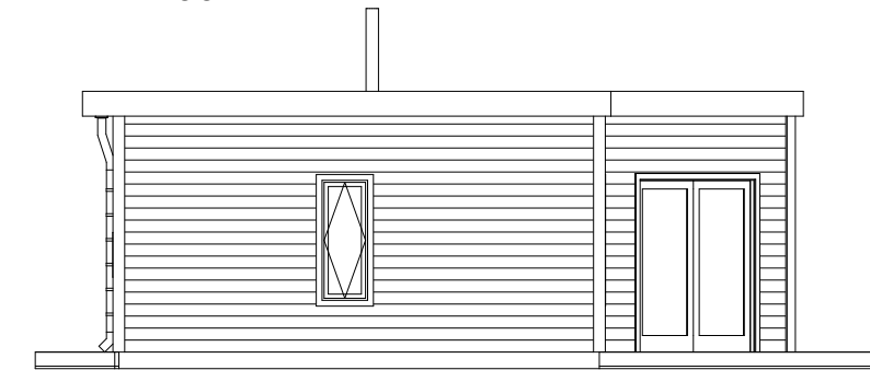
Fasad A4 1:100
