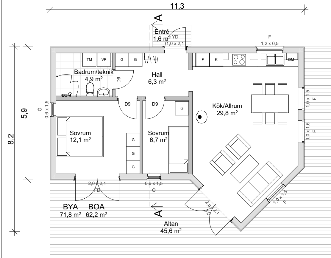
Plan 1 1:100
