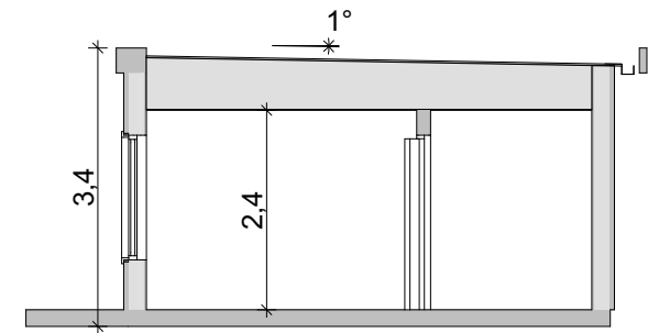
Sektion A 1:100
