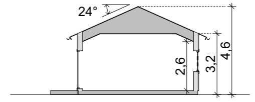
Sektion A 1:200
