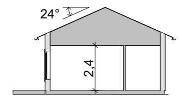
Sektion B 1:200
