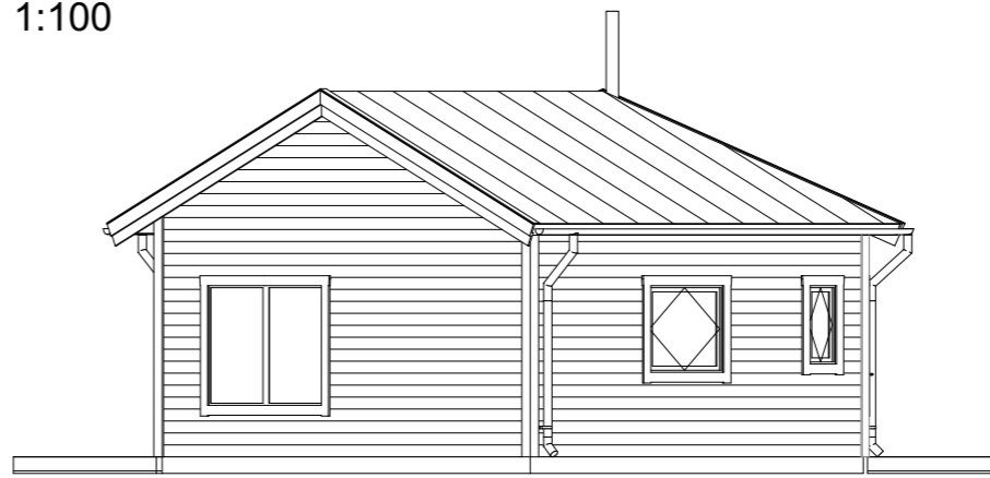
Fasad A4 1:100
