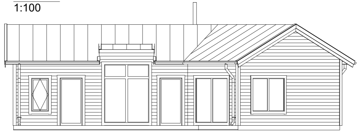
Fasad A3 1:100
