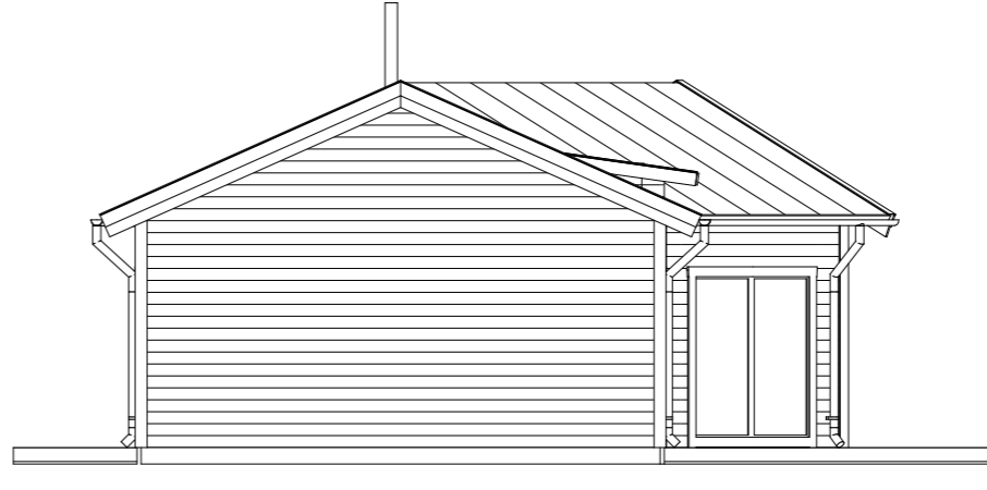
Fasad A2 1:100
