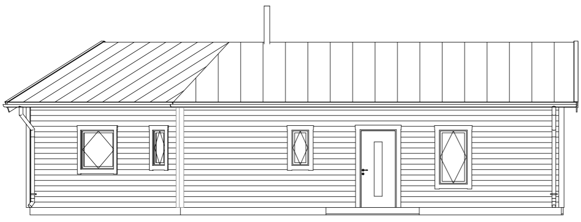
Fasad A1 1:100
