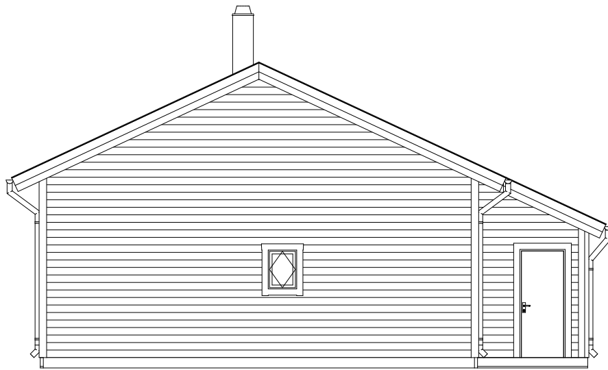
FASAD A4 1:100
