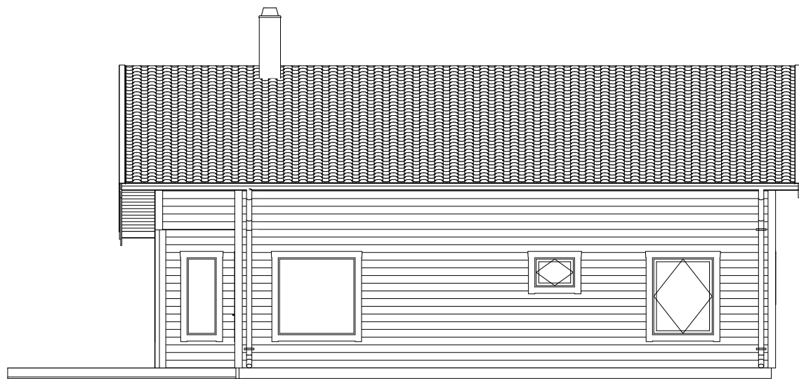
FASAD A3 1:100
