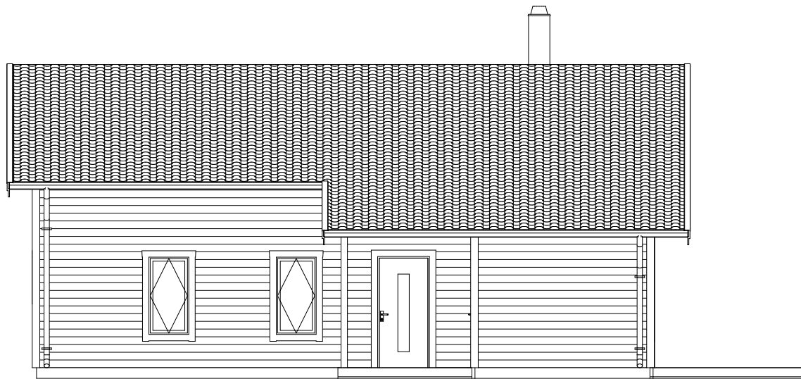
FASAD A1 1:100
