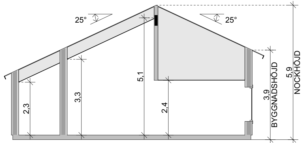
Sektion A 1:100
