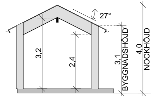
Sektion A 1:100
