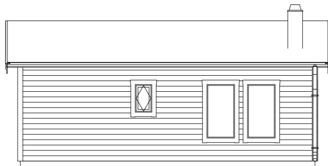
FASAD A1 1:100
