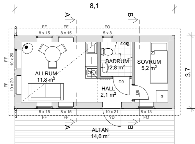
PLAN 1 1:100
