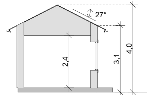
Sektion B 1:100
