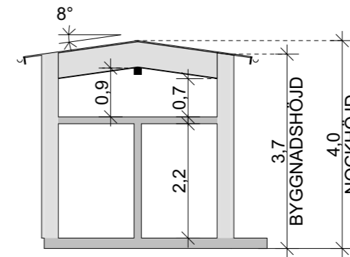
Sektion A 1:100
