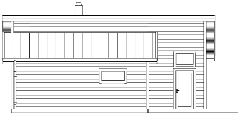
FASAD A3 1:100
