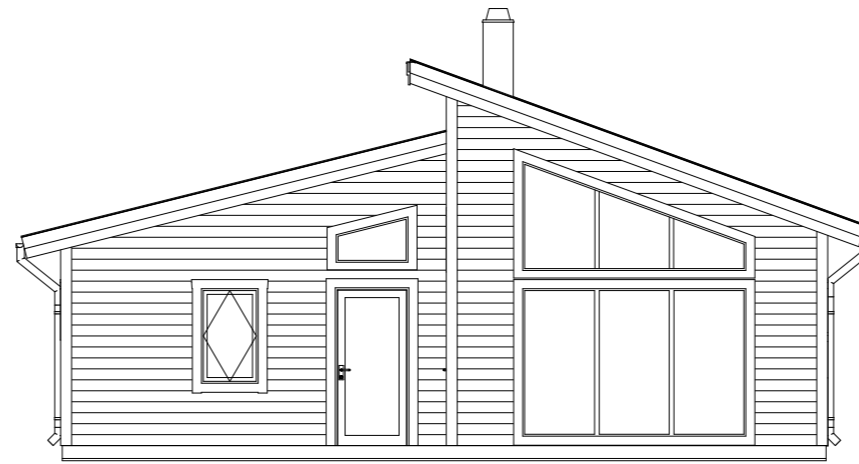
FASAD A4 1:100
