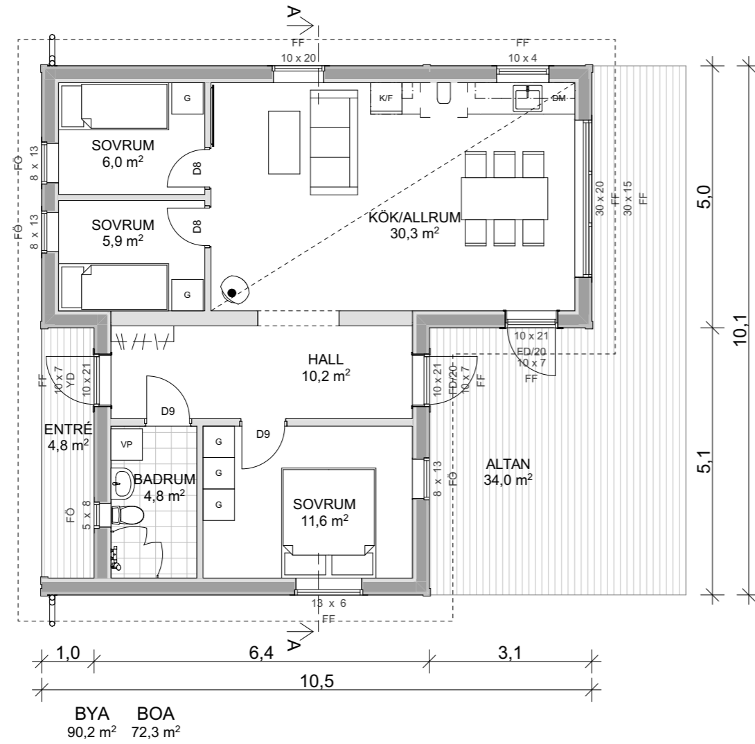
PLAN 1 1:100
