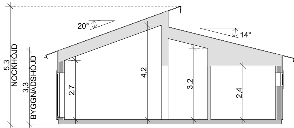
Sektion A-A 1:100
