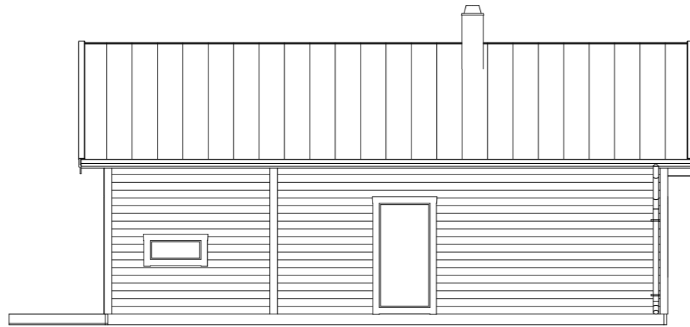
FASAD A1 1:100
