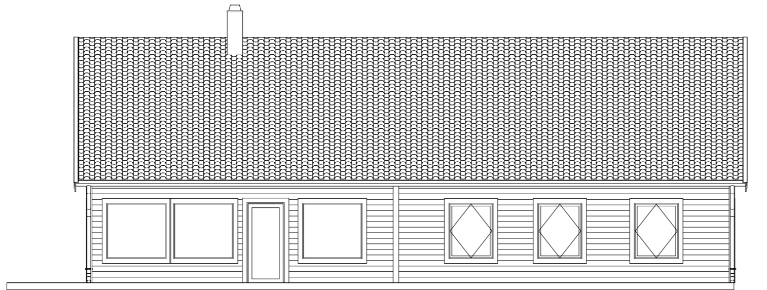
FASAD A1 1:100
