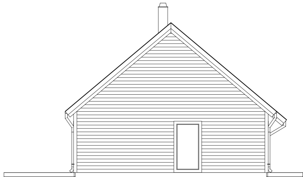
FASAD A2 1:100
