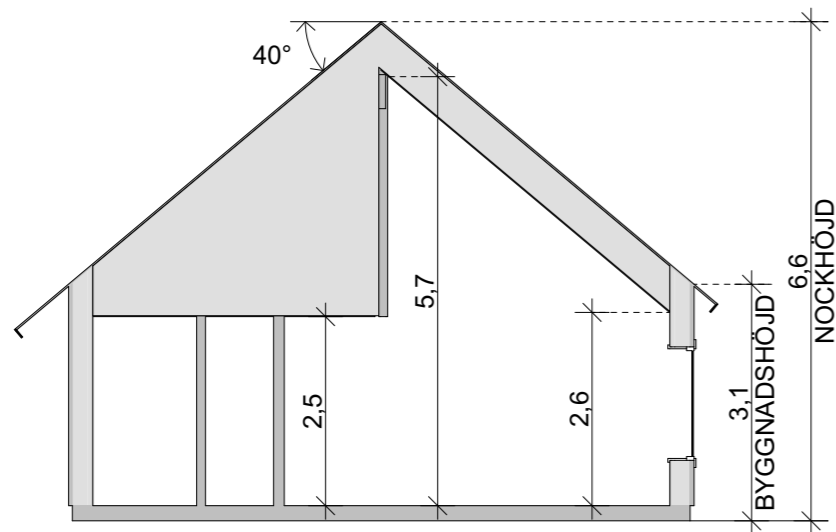
SEKTION A 1:100
