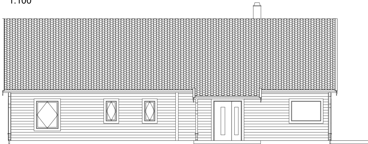
FASAD A3 1:100
